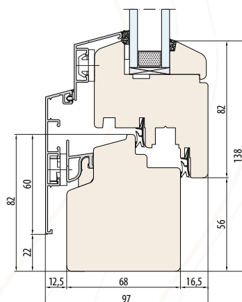
SYSTEM NATURO 68 ALU RENO LINE bez podcięcia pod parapet
