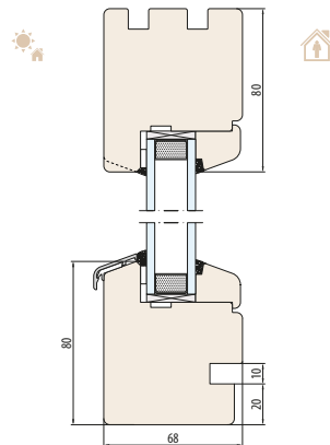
SYSTEM NATURO 68-Fix podcięcie pod parapet wewnętrzne
