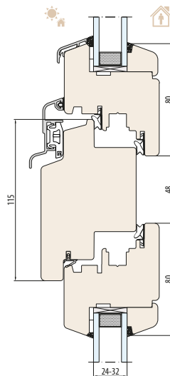
SYSTEM NATURO 68 ślepię 115 mm
