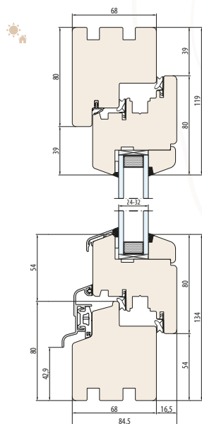
SYSTEM NATURO 68 bez podcięcia pod parapet
