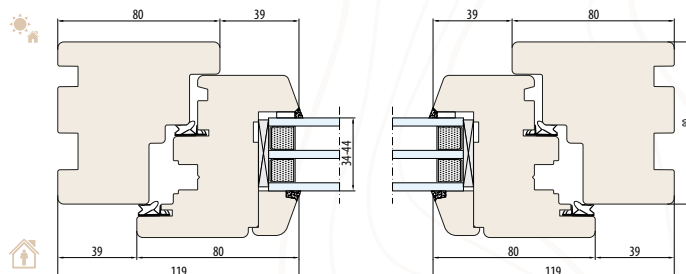
SYSTEM NATURO 80 PRZĘKRÓJ POZIOMY B-B
