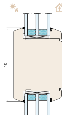
SYSTEM NATURO 92 szpros konstrukcyjny 140 mm
