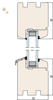
SYSTEM NATURO 68-Fix bez podcięcia pod parapet
