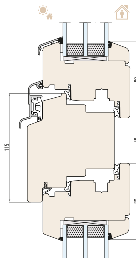
SYSTEM NATURO 92 ślemię 115 mm
