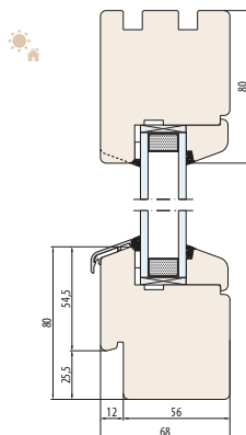
SYSTEM NATURO 68-Fix podcięcie pod parapet zewnętrzne
