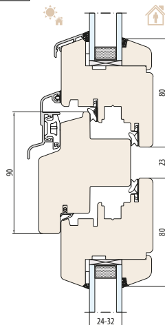
SYSTEM NATURO 68 ślepię 90 mm
