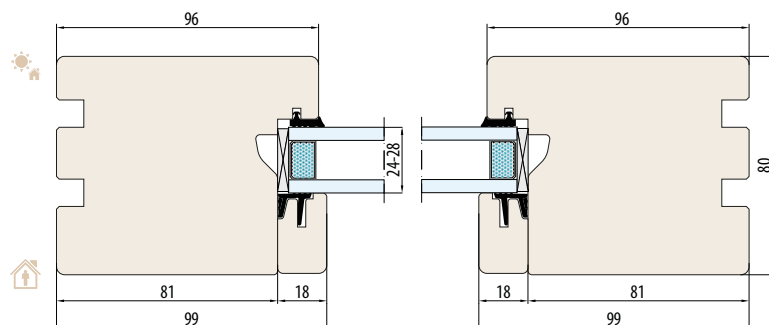
SYSTEM ESPERIA LIFE 80-Fix PRZĘKRÓJ POZIOMY B-B
