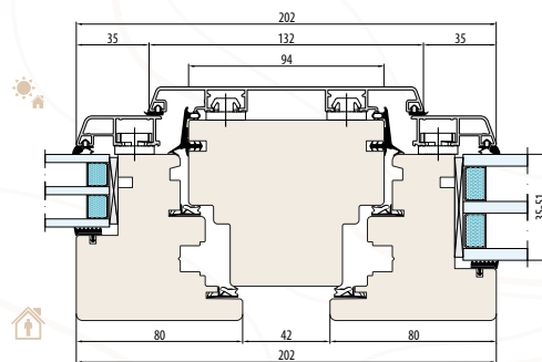
słupki stały 94 mm (przekrój poziomy)
