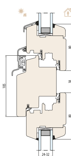
SYSTEM NATURO 68 ślepię 105 mm
